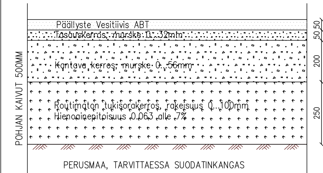
DET 1. RAKENNEKERROKSET
